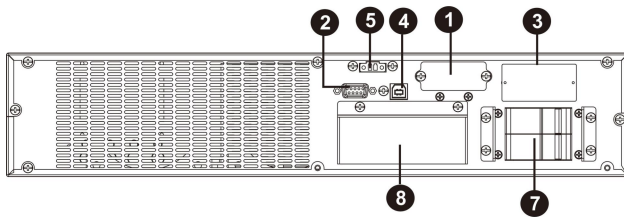
图 4: 6KR(L) 背面面板
