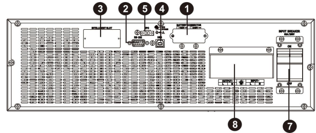
图 5: 10KR(L) 背面面板
